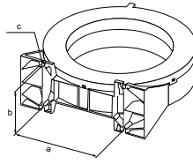
CTBC120(P)/CTBC210(P)
